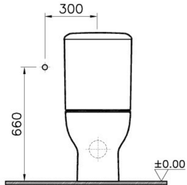
Yandan girisli Side inlet Zulauf seitlich
