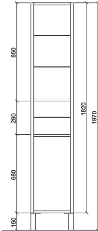
Nárys
