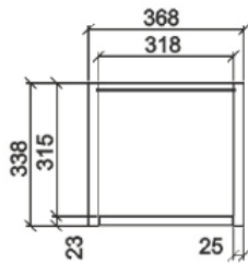
Pűdorys
